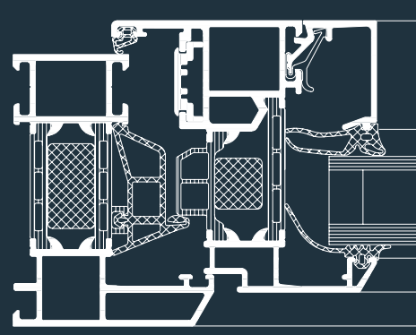
Schüco Окно AWS 70 RL.HI Масштаб 1:2 Schüco Window AWS 70 RL.HI Scale 1:2
