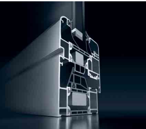
Schüco Окно AWS 70 SL.HI Закругленный контур створок для создания более плавных линий Schüco window AWS 70 SL.HI Rounded Soft Line vent contour for soft lines
