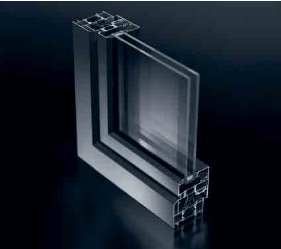
Schüco Окно AWS 65 RL Система со скошен. внешн. контурами Schüco window AWS 65 RL System with bevelled exterior contour
