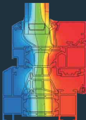
Schüco окно AWS 70 RL.HI Сокращение энергопотерь Schüco window AWS 70 RL.HI Reduced heat loss
