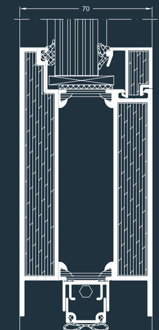
Дверь Schüco Firestop II EI60, Вертикальное сечение Schüco Firestop II EI60 door, vertical section detail
