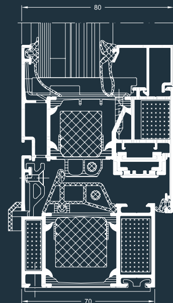
Schüco Окно AWS 70 FR 30 Вертикальное сечение Schüco Window AWS 70 FR 30 Vertical section detail
