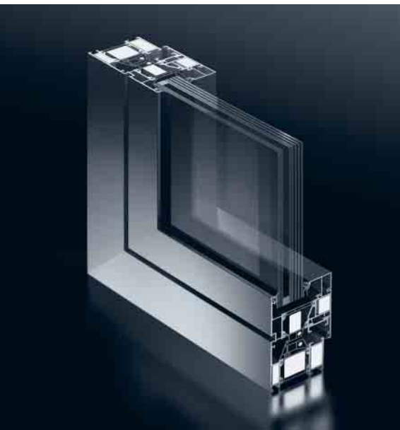
Schüco Окно AWS 70 FR 30 Вертикальное сечение Schüco Window AWS 70 FR 30 Vertical section detail
