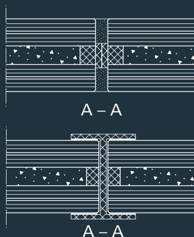
Schüco Firestop II F30 PG Силиконовый шов и H-профиль, горизонтальное сечение Silicone joint and H-shaped profile, horizontal section detail
