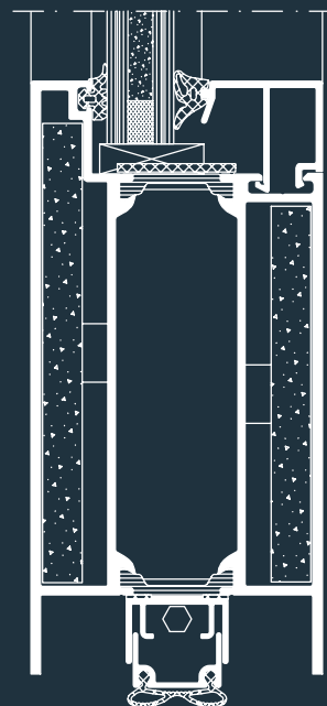
Schüco Firestop II, дверь T30 изнутри вертикальное сечение Schüco Firestop II, T30 door inside Vertical section detail
